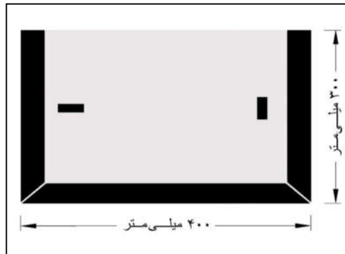
شکل ۱۲: تابلوی کشویی غلاف دار نوع دوم
