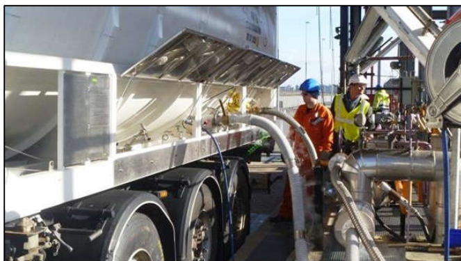
شکل ۴: قرار گرفتن تجهیزات بارگیری و تخلیه تانکرهای قابل حمل در محفظه ای محفوظ
