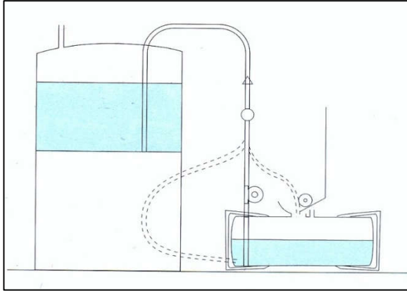
شکل ۲۵: تخلیه با پمپاژ
