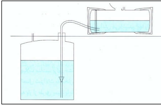
شکل ۲۴: تخلیه ثقلی
